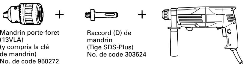
Clé de mandrin
